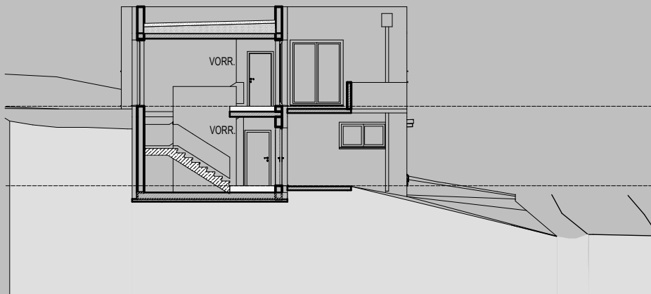
SCHNITT A-A
