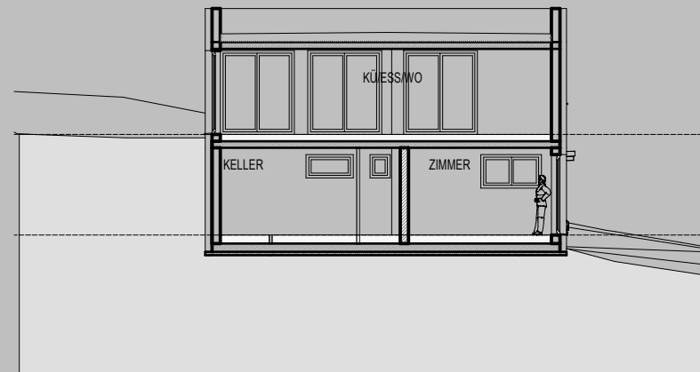
SCHNITT B-B
