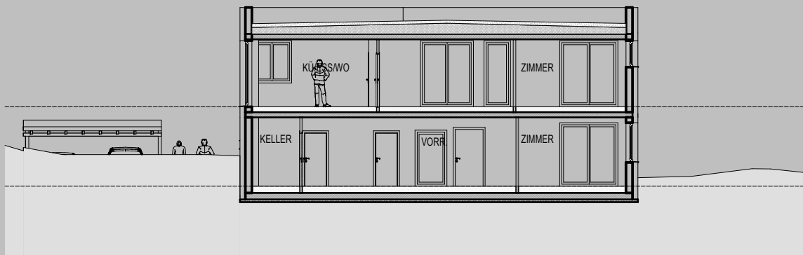
SCHNITT C-C
