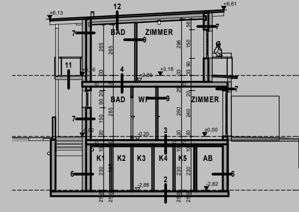
SCHNITT C-C
