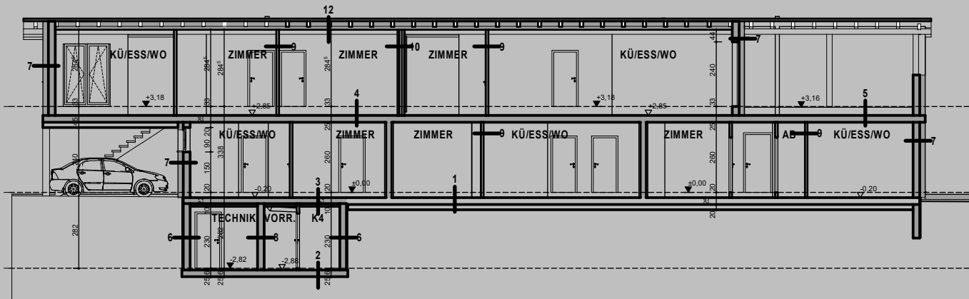
SCHNITT A-A
