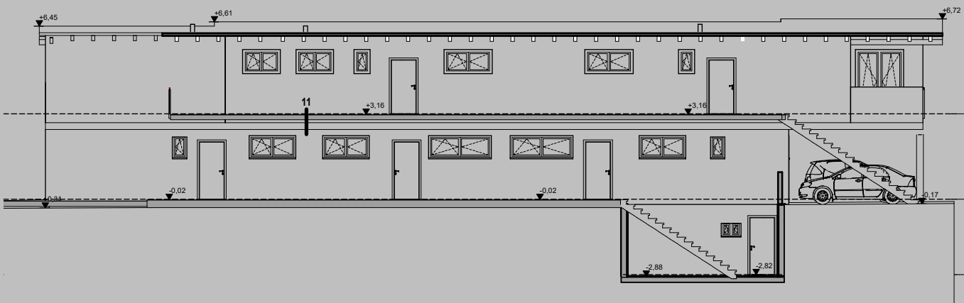
SCHNITT B-B
