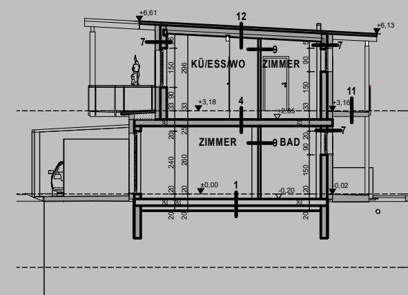
SCHNITT D-D
